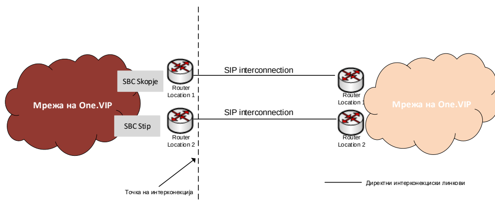
Слика 4. SIP Сигнално поврзување помеѓу мрежите на двете Страни.
