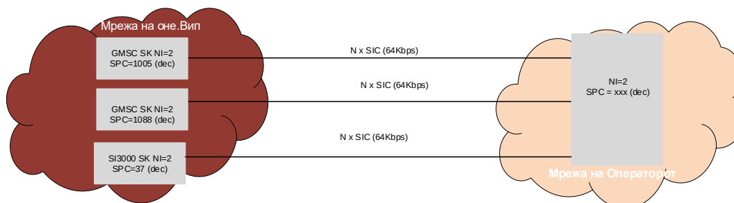
Слика 3. TDM Сигнално поврзување помеѓу мрежите на двете Страни.
