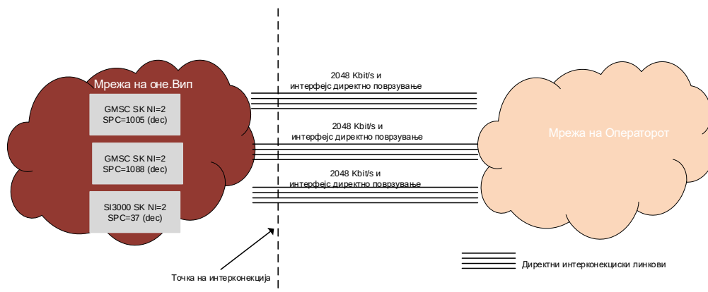
Слика 1. Приказ на TDM Интерконекцијата
